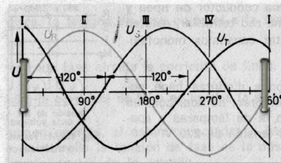
DIAGRAMA ELÈCTRIC TRIFÀSIC
